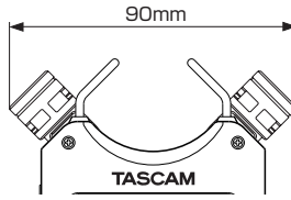
Размеры с микрофонами в раскрытом положении
