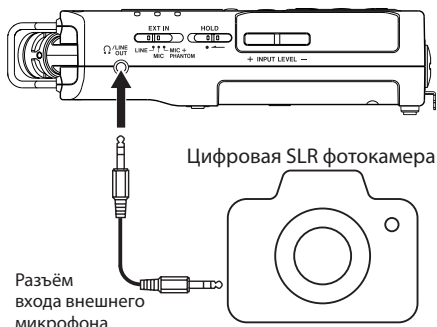
Пример подключения
